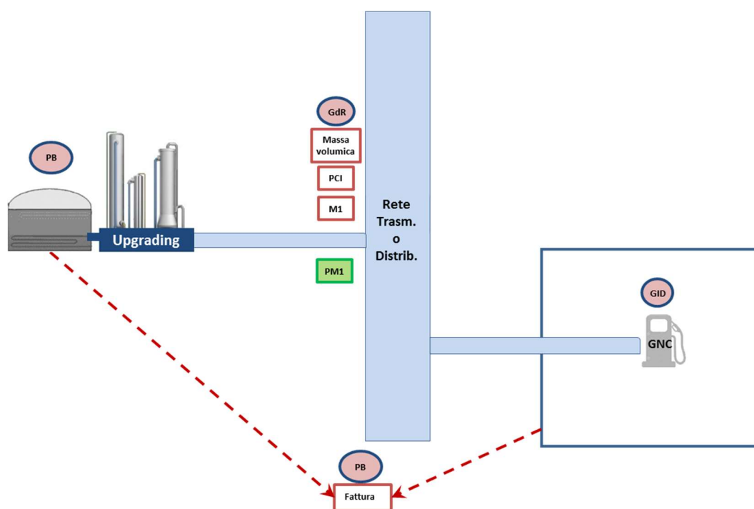
Figura 7 – Schema dei punti di misura e delle grandezze rilevanti ai fini del calcolo della quantità ammessa all'incentivo nel caso di immissione in consumo nei trasporti mediante reti con obbligo di connessione di terzi senza il ritiro del biometano.
