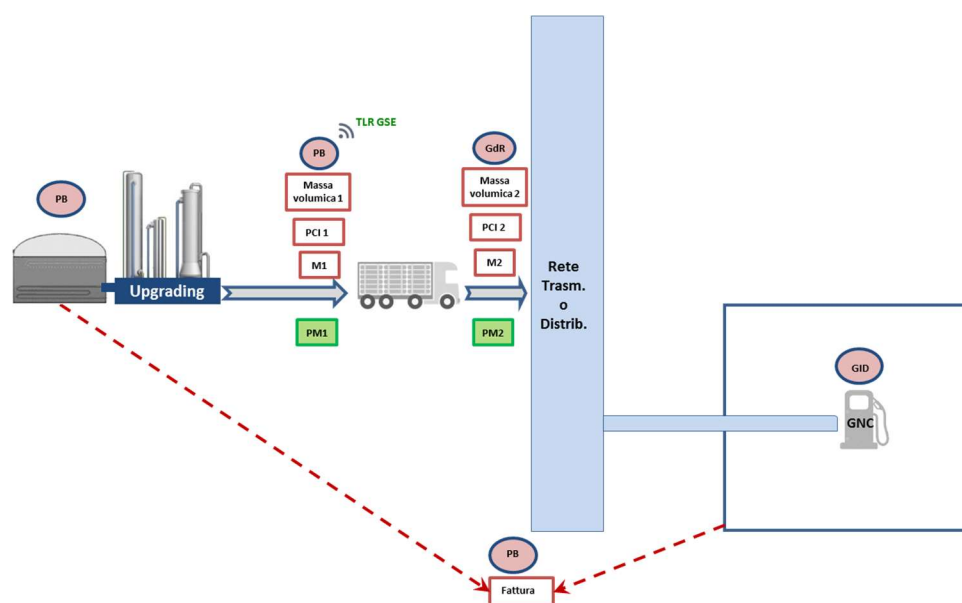
Figura 8 – Schema dei punti di misura e delle grandezze rilevanti ai fini del calcolo della quantità ammessa all’incentivo nel caso di immissione in consumo nei trasporti mediante rete con obbligo di connessione di terzi collegata all’impianto di produzione tramite carri bombolai, senza il ritiro del biometano.
