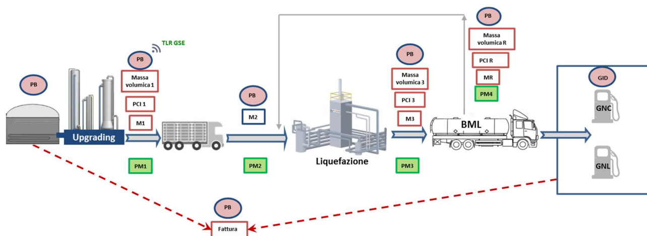
Figura 14 – Schema dei punti di misura e delle grandezze rilevanti ai fini del calcolo della quantità ammessa all’incentivo nel caso di immissione in consumo mediante il trasporto del biometano in forma liquida (BML) e connessione all’impianto di liquefazione tramite carri bombolai, senza ritiro del biometano.
