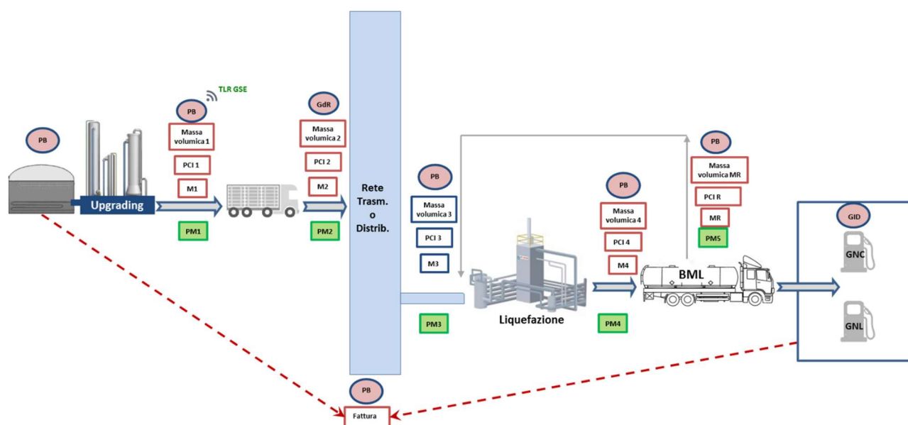
Figura 16 – Schema dei punti di misura e delle grandezze rilevanti ai fini del calcolo della quantità ammessa all’incentivo nel caso di immissione in consumo mediante il trasporto del biometano in forma liquida (BML) e connessione all’impianto di liquefazione tramite rete con obbligo di connessione di terzi connessa all’impianto di produzione tramite carri bombolai, senza ritiro del biometano.
