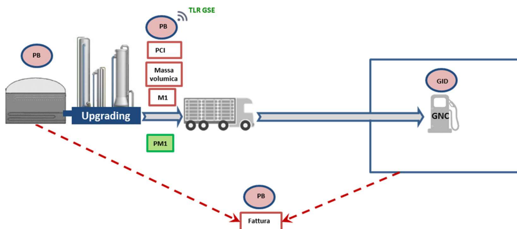
Figura 10 – Schema dei punti di misura e delle grandezze rilevanti ai fini del calcolo della quantità ammessa all’incentivo nel caso di immissione in consumo nei trasporti mediante carri bombolai, senza il ritiro del biometano.
