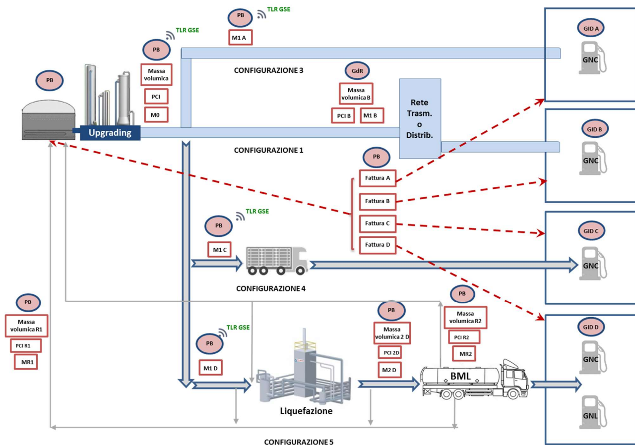
Figura 19 – Schema dei punti di misura e delle grandezze rilevanti ai fini del calcolo della quantità ammessa all’incentivo nel caso di immissione in consumo nei trasporti mediante modalità di trasporto del biometano ibride.
