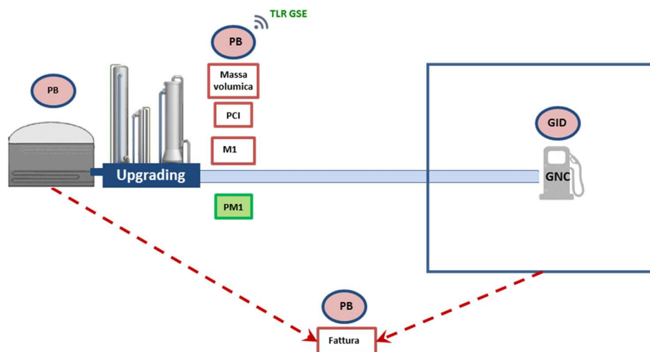
Figura 9 – Schema dei punti di misura e delle grandezze rilevanti ai fini del calcolo della quantità ammessa all'incentivo nel caso di immissione in consumo nei trasporti mediante connessione diretta all'impianto di distribuzione di gas naturale senza ritiro del biometano.
