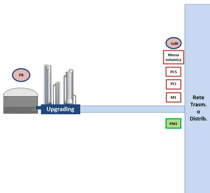
Figura 17 – Schema dei punti di misura e delle grandezze rilevanti ai fini del calcolo dei corrispettivi per il ritiro e della quantità ammessa all’incentivo nel caso di ritiro del biometano immesso nelle reti con obbligo di connessione di terzi.
