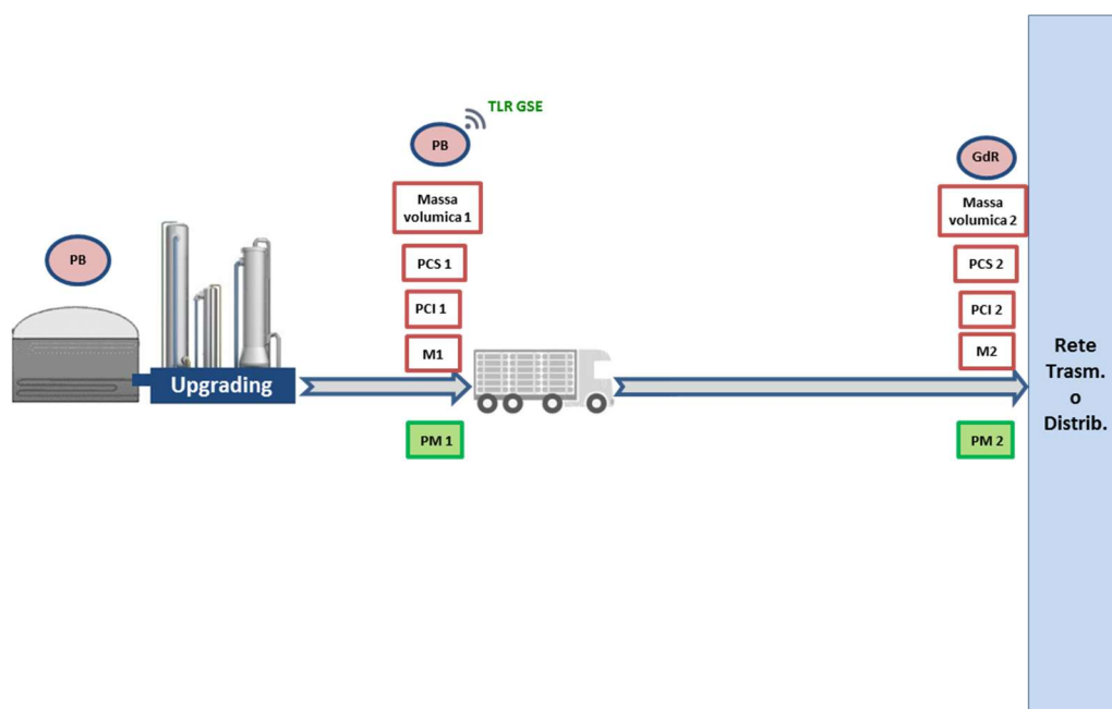
Figura 18 – Schema dei punti di misura e delle grandezze rilevanti ai fini del calcolo dei corrispettivi di ritiro e della quantità ammessa all’incentivo nel caso di ritiro del biometano immesso nelle reti con obbligo di connessione di terzi tramite carri bombolai.
