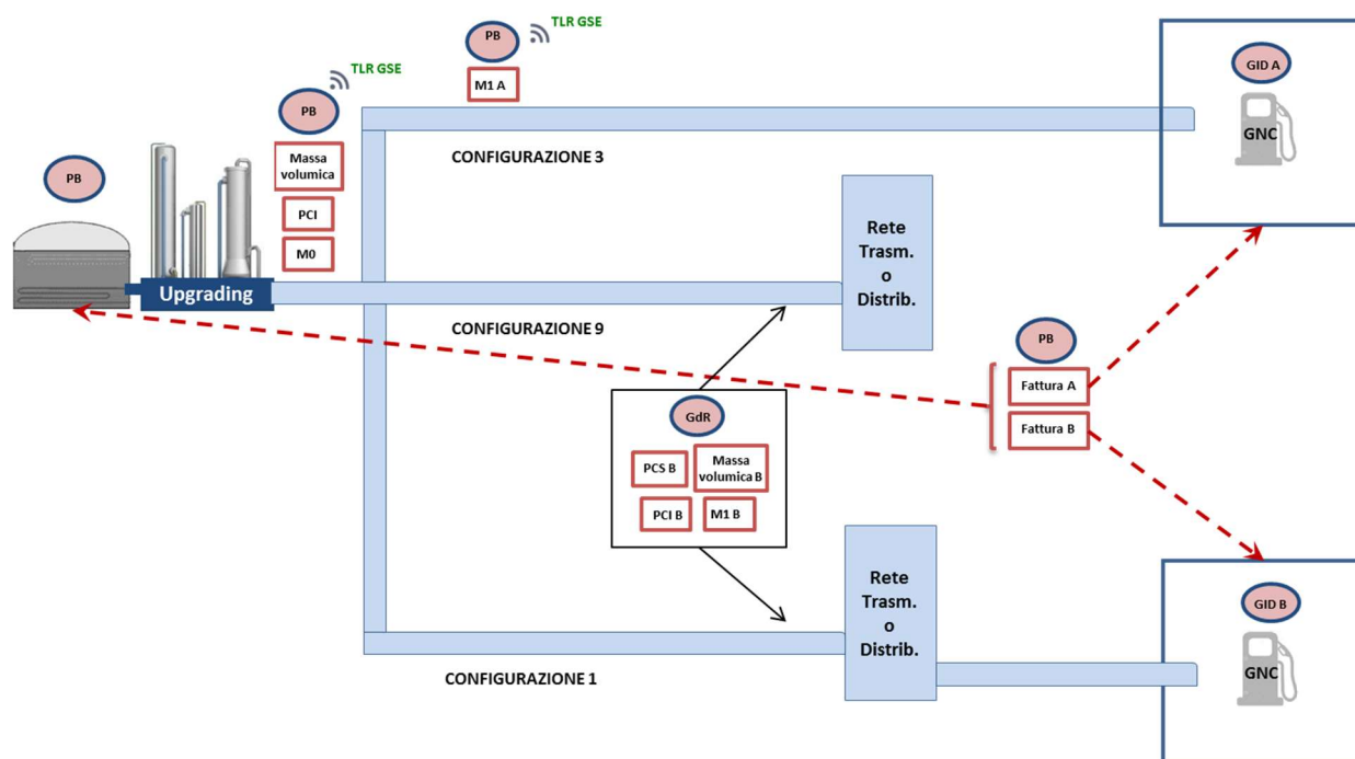
Figura 20 – Schema dei punti di misura e delle grandezze rilevanti ai fini del calcolo della quantità ammessa all’incentivo nel caso di ritiro parziale del biometano.
