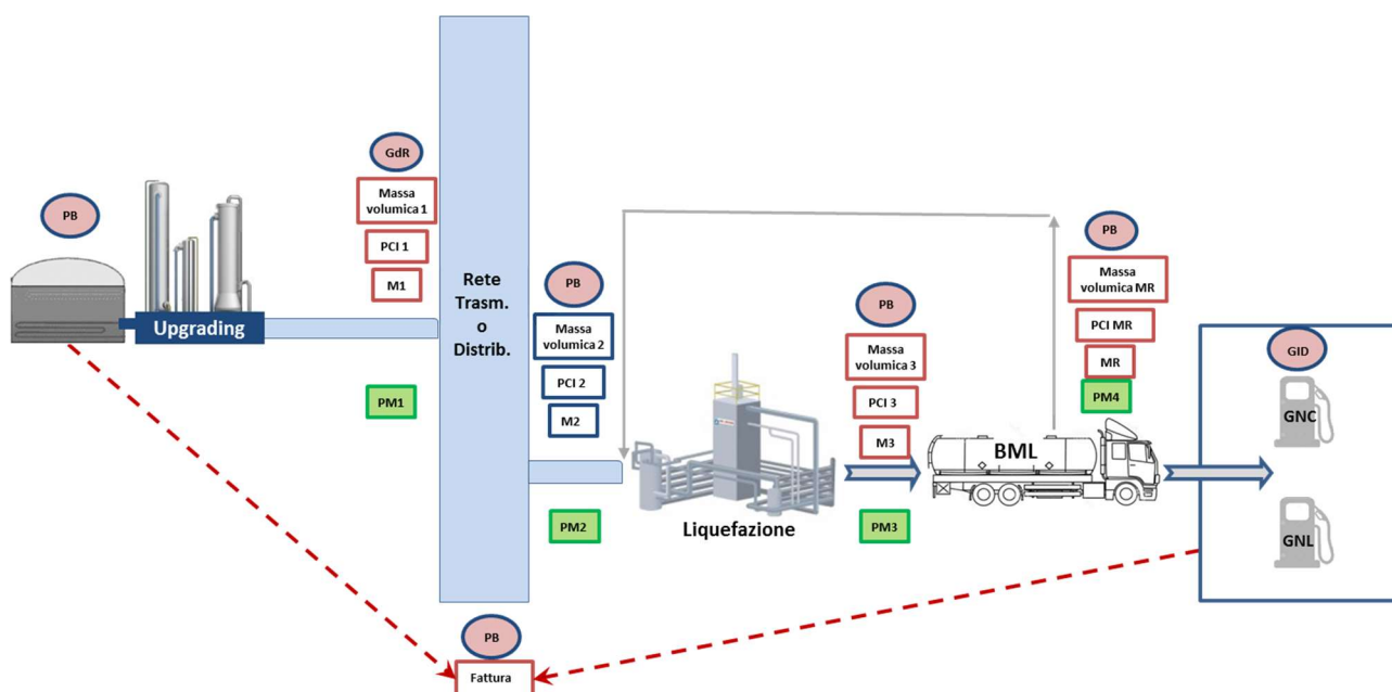
Figura 15 – Schema dei punti di misura e delle grandezze rilevanti ai fini del calcolo della quantità ammessa all'incentivo nel caso di immissione in consumo mediante il trasporto del biometano in forma liquida (BML) e connessione all'impianto di liquefazione tramite rete con obbligo di connessione di terzi, senza ritiro del biometano.
