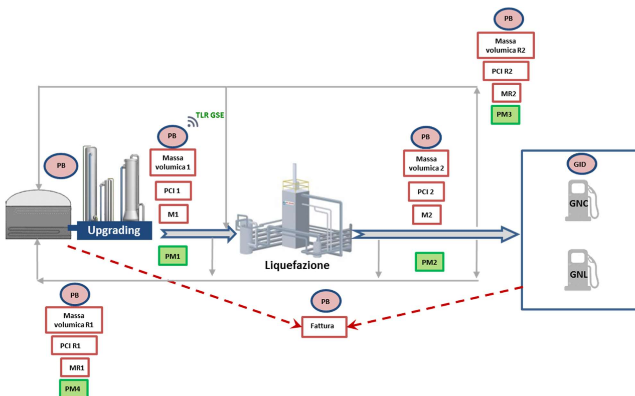
Figura 13 – Schema dei punti di misura e delle grandezze rilevanti ai fini del calcolo della quantità ammessa all'incentivo nel caso di immissione in consumo del biometano in forma liquida (BML) tramite connessione diretta all'impianto di liquefazione e a quello di distribuzione, senza ritiro del biometano da parte del GSE.
